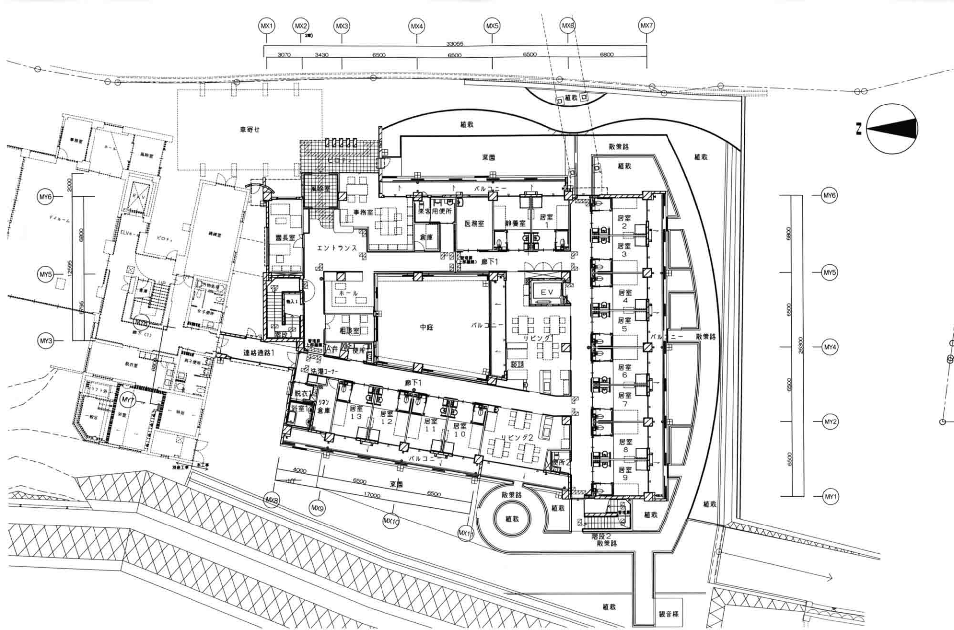
配置図兼1階平面図
